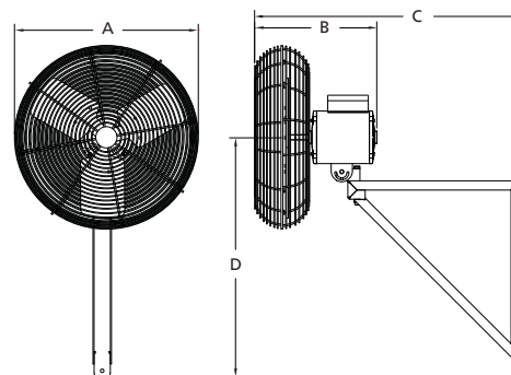
Figure 6 — Dimensions du 3PEH2
