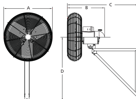
Figura 3 — Dimensiones 3PEG9
