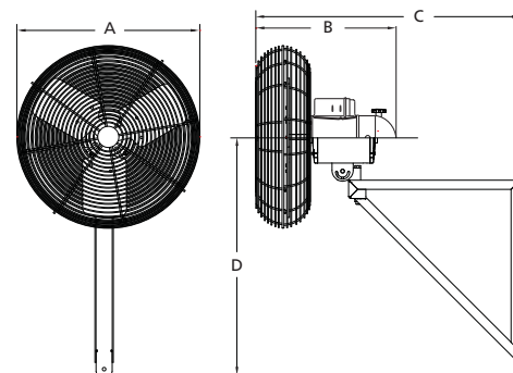
Figure 3 — Dimensions du 3PEG9
