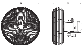
Figura 2 — Dimensiones Giratorias
