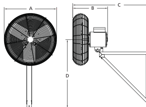
Figura 6 — Dimensiones de los Modelos 3PEH2
